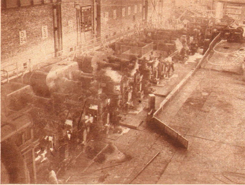
Una vista del tren de laminación Morgan, en funcionamiento en la planta de Villa Constitución.
