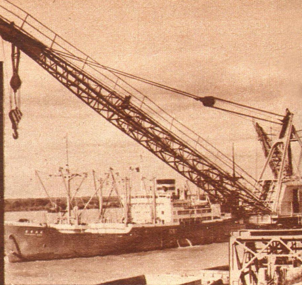
Una de las dos poderosas grúas Colby, de 45 toneladas de capacidad, que funcionan en el puerto propio de Acindar, en V. Constitución.
