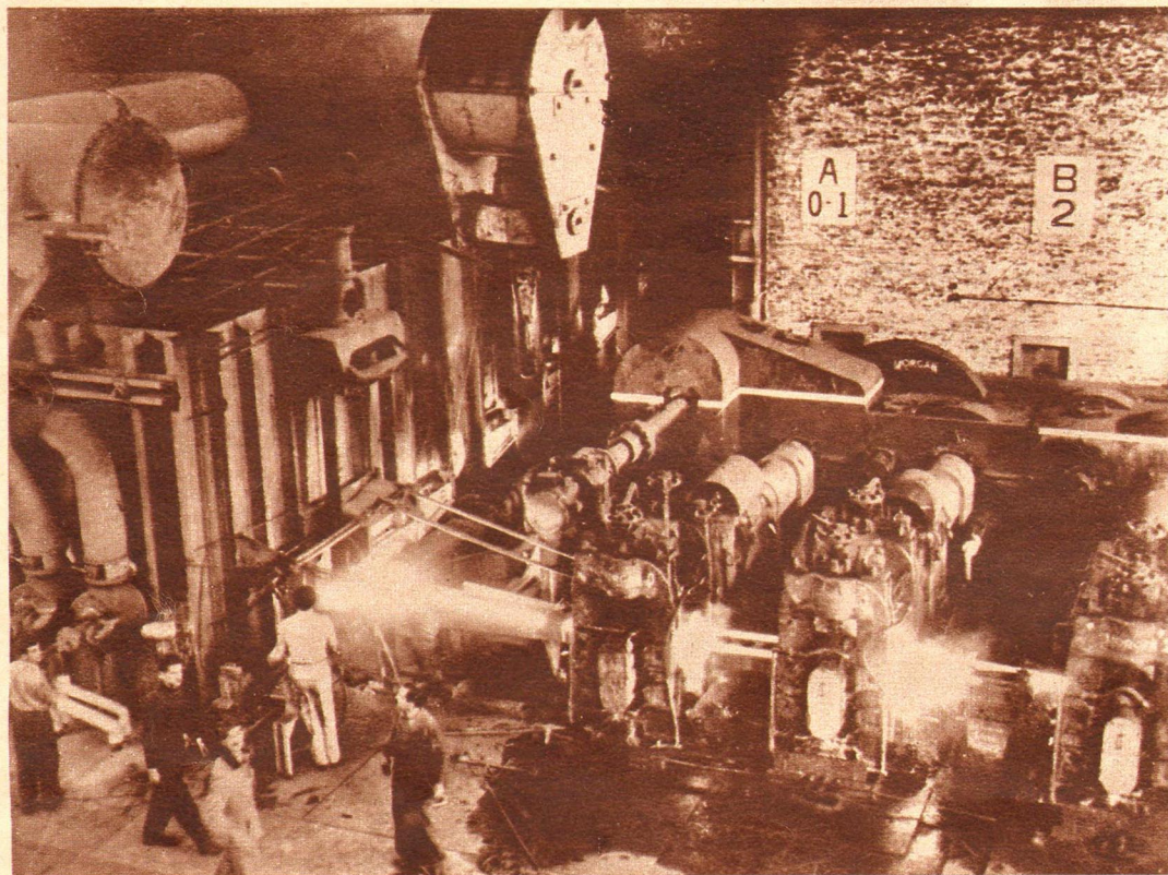
El horno de calentamiento de palanquillas y vista parcial del tren de laminación Morgan.
