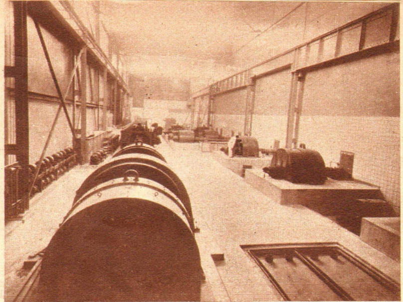
Detalle de un sector de la sata de motores, existente en la planta de Villa Constitución, provincia de Santa Fe
